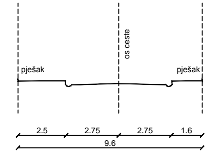
KARAKTERISTIČAN POPREČNI PRESJEK C - C, MJ. 1:200
