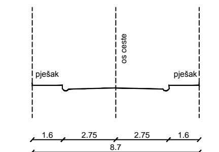
KARAKTERISTIČAN POPREČNI PRESJEK D - D, MJ. 1:200
